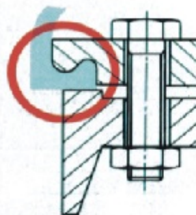
falsche Montage
