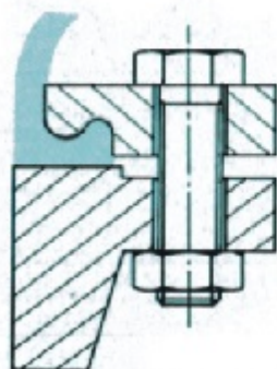
richtige Montage
